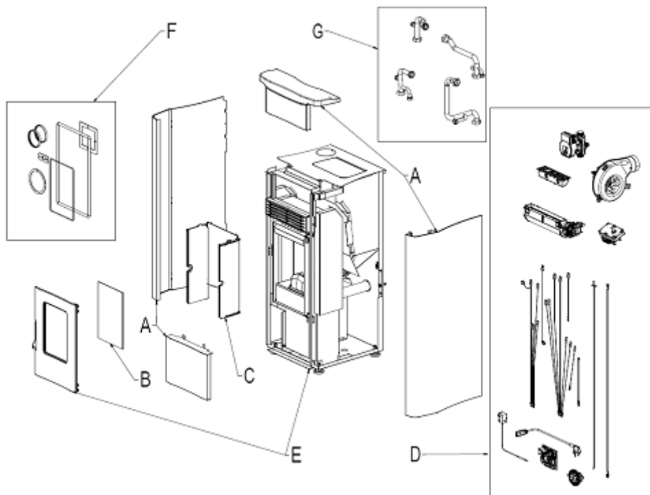
Fig. 1 - Geëxploedeerde tekening
