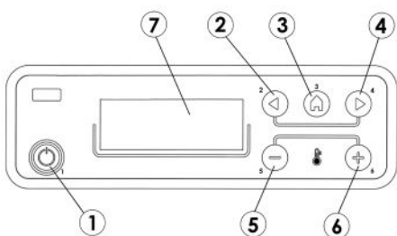
Fig. 8 - Bedieningspaneel
