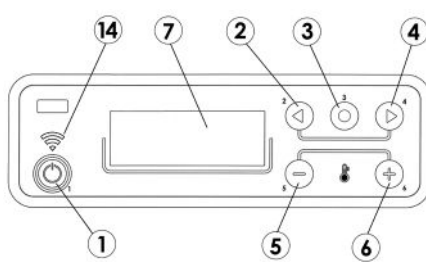
Fig. 9 - Bedieningspaneel (wi-fi)
