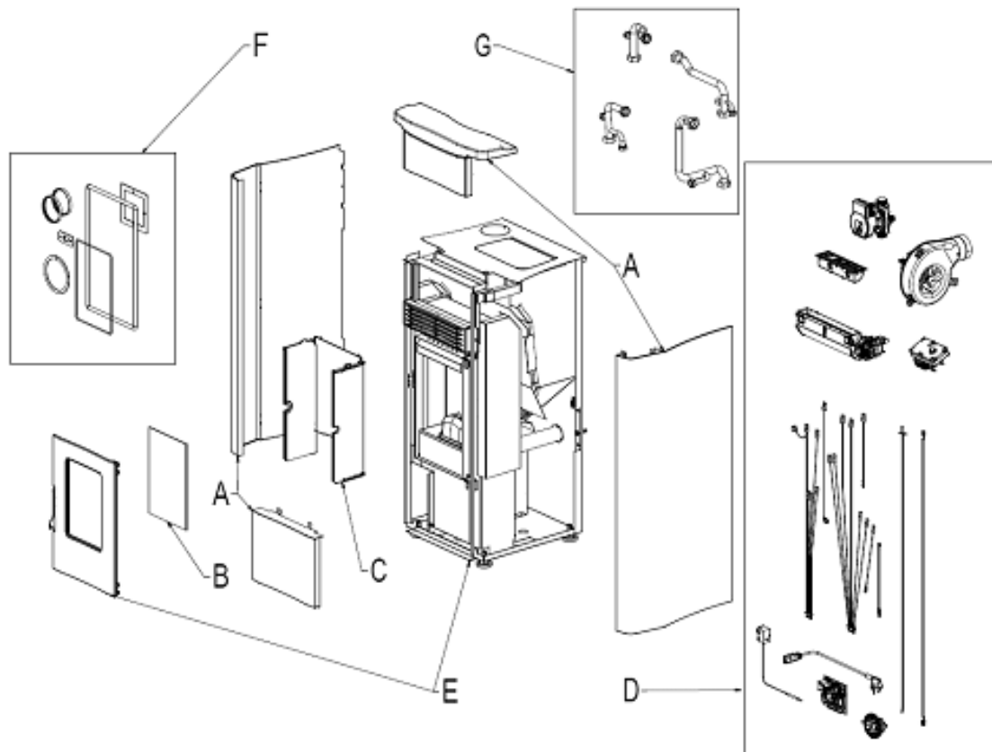
Fig. 1 - Geëxplodeerde tekening
