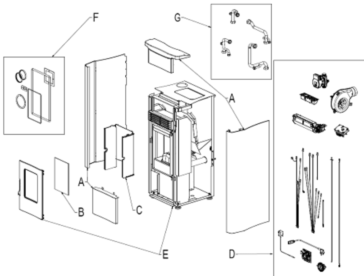
Fig. 1 - Geëxplodeerde tekening
